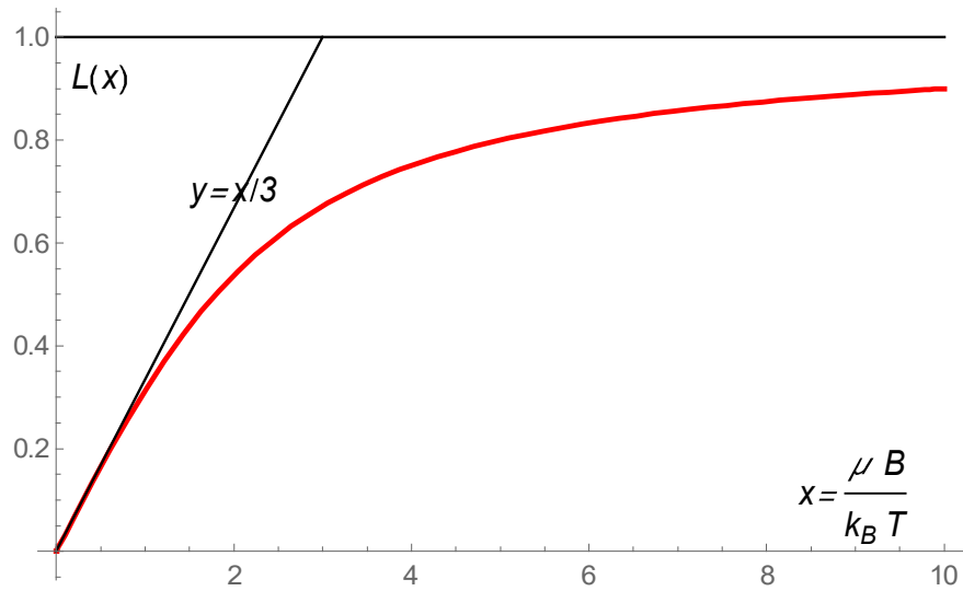
Fig. Langevin function L(x) .
