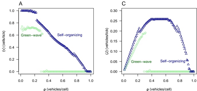
Figure: Resultados para una malla 10x10: (A) velocidad promedio \langle v \rangle y (C) flujo promedio \langle J \rangle para distintas densidades \rho .
