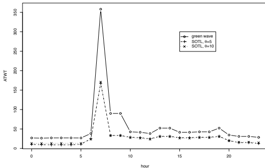
Figure: Tiempos de espera por viaje promedio (ATWT) para distintas horas del día laboral.
